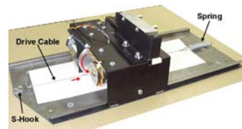
T-3918 Sled Assembly
